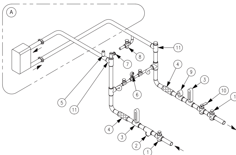
Рис. 23 - Рекомендуемый трубопровод конденсатора для типового испарителя RTAD без трехходового клапана
