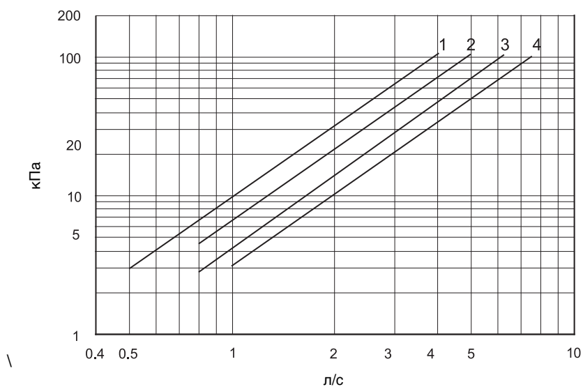
Рис. 15 - Падение давления на конденсаторе RTAD с частичной рекуперацией тепла - режим нагрева
